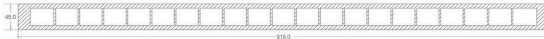
木塑门扇 45 厚 CAD
